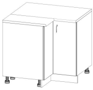
11 прав 900*900*850
