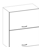
вг 60/72 600*320*720
