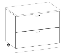
№ 4 ш2 (100) 1000*600*850
