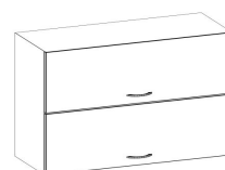
вг 90/60 900*320*600
