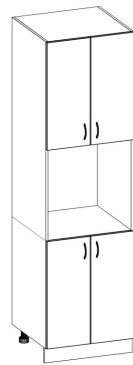
48 (60) 713/600н/713 600*580*2140
