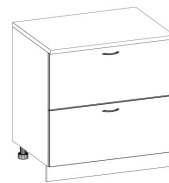
№ 4 ш2 (80) 800*600*850
