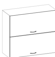
вг 80/72 800*320*720
