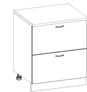
№ 4 ш2 (70) 700*600*850
