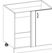
2у прав 800*600*850
