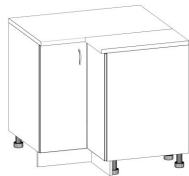
11 лев 900*900*850
