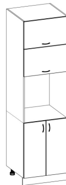
48 (60) 355/355/600н/713 600*580*2140
