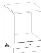
гп + дш 600*600*850
