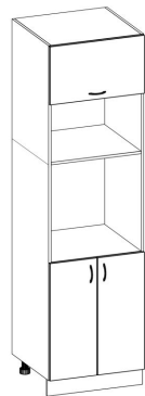
48 (60) 355/360н/600н/713 600*580*2140
