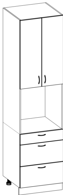
пенал 48(60В) [913/600Н/Ш3] выс./шир./глуб. 2340/600/580
