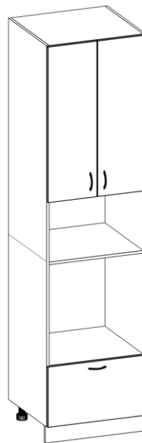
пенал 48(60В) [913/360Н/600Н/Ш1] выс./шир./глуб. 2340/600/580
