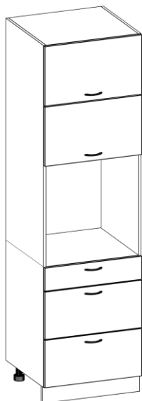
пенал 48(60) [355/355/600Н/Ш3] выс./шир./глуб. 2140/600/580
