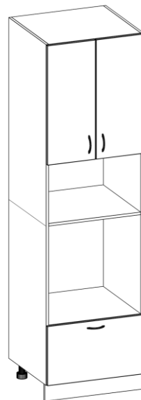
пенал 48(60) [713/360Н/600Н/Ш1] выс./шир./глуб. 2140/600/580
