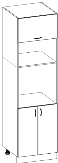
пенал 48(60) [355/360Н/600Н/713] выс./шир./глуб. 2140/600/580
