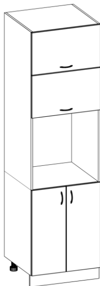
пенал 48(60) [355/355/600Н/713] выс./шир./глуб. 2140/600/580
