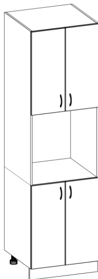
пенал 48(60) [713/600Н/713] выс./шир./глуб. 2140/600/580
