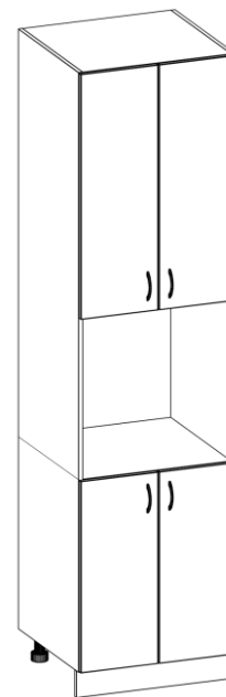
пенал 48(60В) [913/600Н/713] выс./шир./глуб. 2340/600/580
