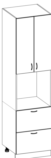
пенал 48(60В) [913/600Н/Ш2] выс./шир./глуб. 2340/600/580
